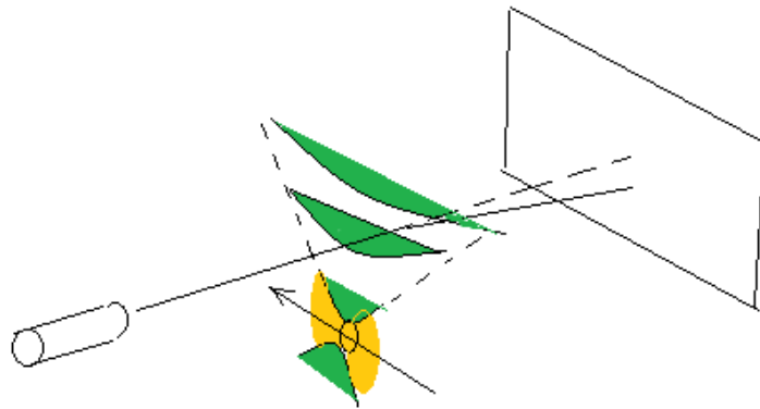
Рис . 4.1. Квантовый гравитация поля .
