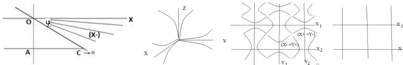
Рисунок 1. Динамичное пространство-материя.
