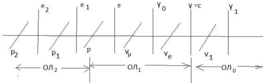
Рисунок 3.1 неделимые кванты пространства-материи.
