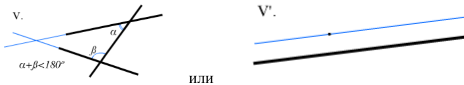
рис. 1 Евклидова аксиоматика
