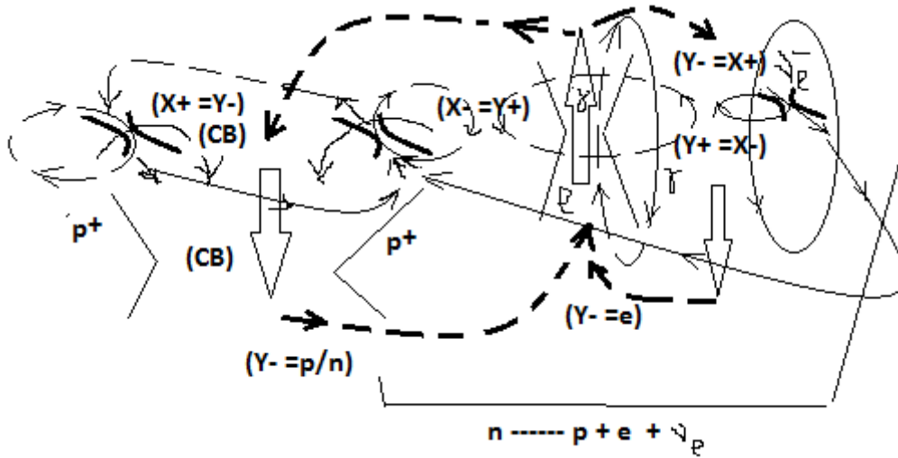
Рисунок.3.6. Квант (Y_{-} = p/n) и аналогично (Y_{-} = 2n) Сильного Взаимодействия Протон здесь, имеет форму тора. Аналогично для электрона, электрическое поле состоит из виртуальных (\gamma) фотонов.
