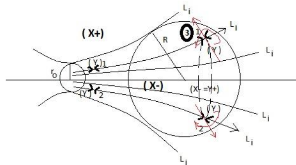
Рис. 3. Модель запутанных частиц.
