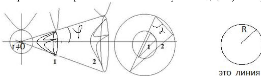
Рисунок 1.2 Изотропная динамика.
