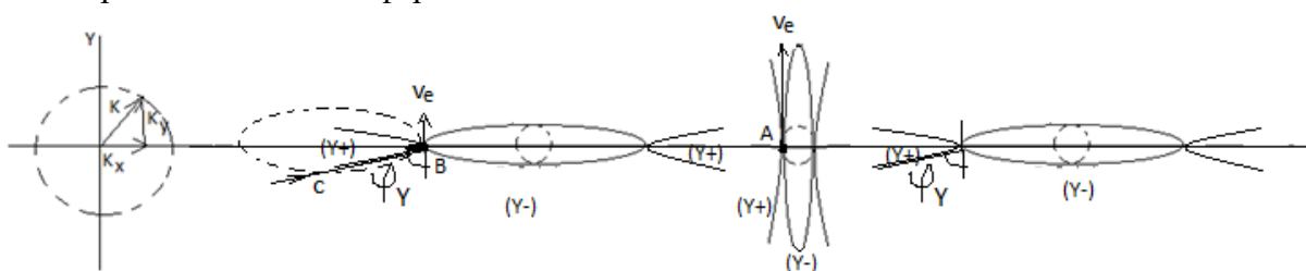
Рисунок 3.1. квантовая релятивистская динамика пространства-материи электрона
