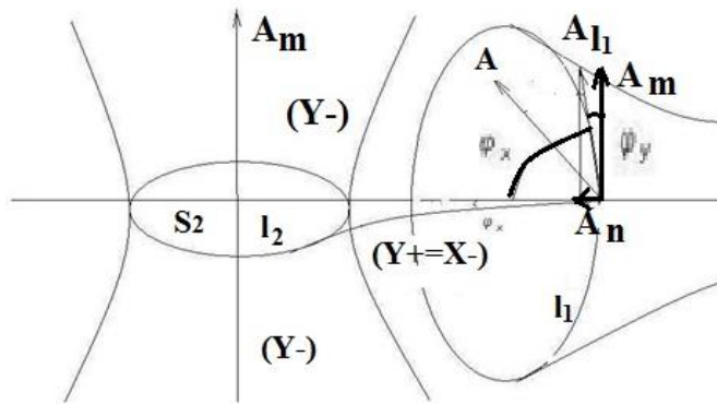
Рисунок 3. Электро ( Y+ = X- ) магнитные и гравит( X+ = Y- ) массовые поля.
