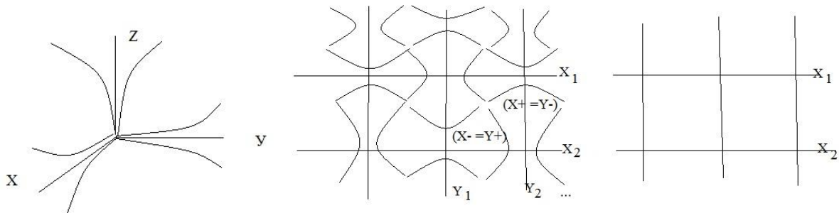
рисунок.3.3 динамичное пространство-материя
