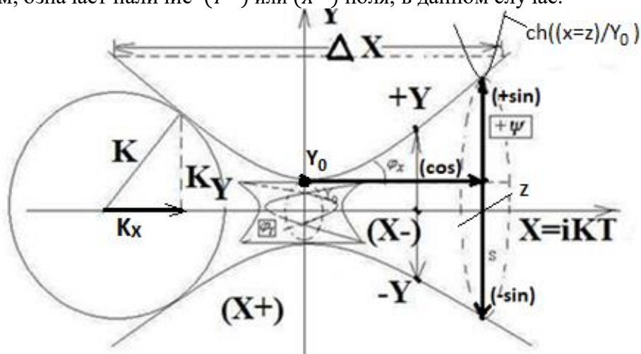
Рисунок 3. Квант (X\pm) динамичного пространства-материи.
