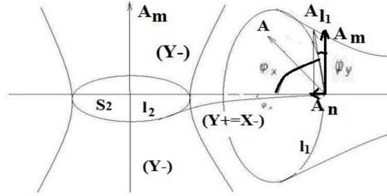
Рисунок 2.2-1. электро (Y+=X-) магнитные и гравит (X+=Y-) массовые поля.
