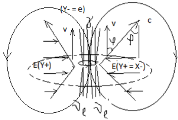
Рисунок 3.5. модель электрона.
