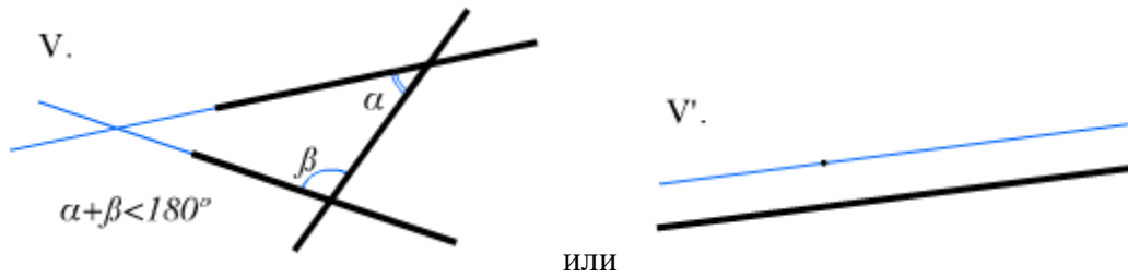
рис. 1 Евклидова аксиоматика
