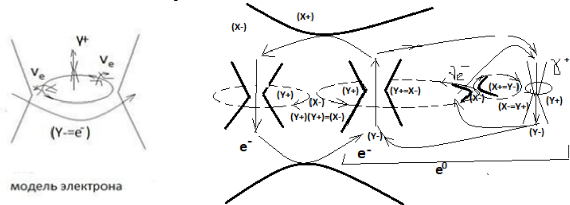
Рисунок 9. Допустимые структуры лептонов.
