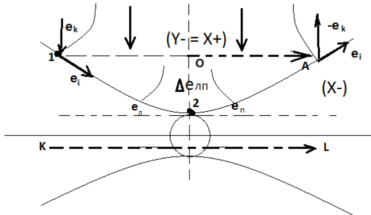
Рисунок 6. Квант пространства-материи
