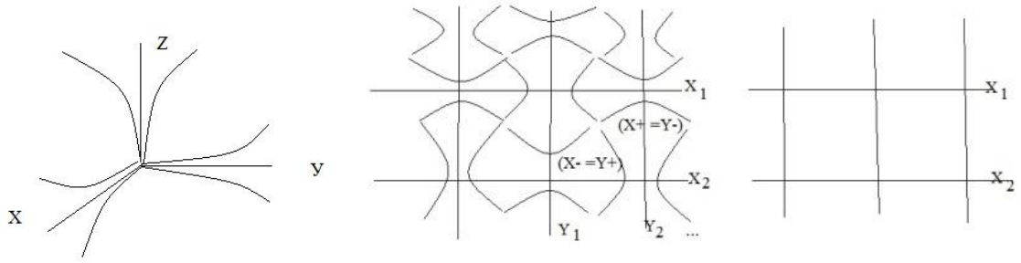
Рис. 1. Динамическое пространство-материя.
