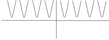
Рисунок 3.3. график динамики квантовых полей
