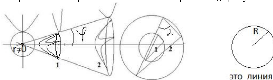
Рисунок 1.2 Изотропная динамика.
