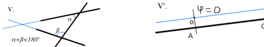
рис. 1 Евклидова аксиоматика.
