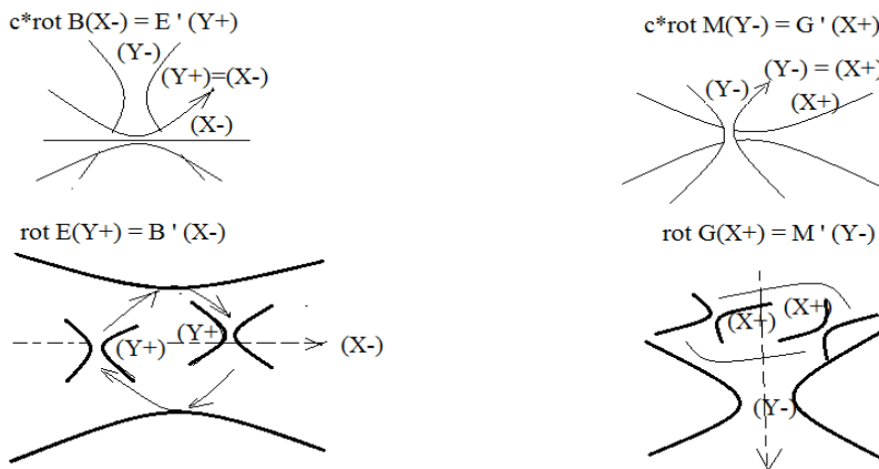
Рисунок 2.2-2. Единые поля пространства-материи
