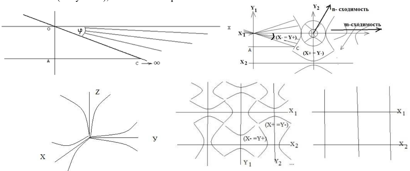
Рисунок 1. Динамичное пространство-материя.
