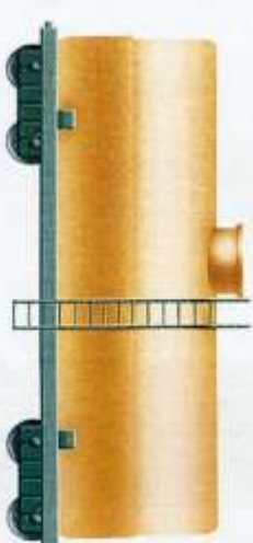
ЦИСТЕРНА ДЛЯ НЕФТЕПРОДУКТОВ (РОССИЯ, ВТОРАЯ ПОЛОВИНА XX в.)
