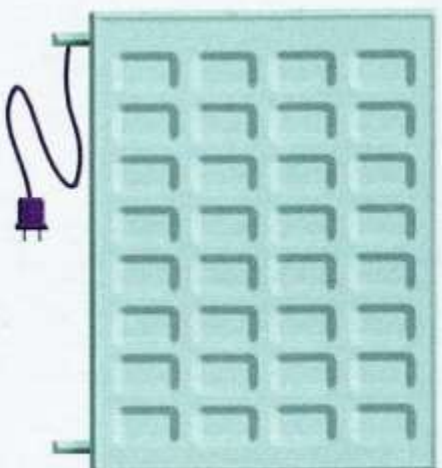
СОВРЕМЕННЫЕ ЭЛЕКТРОНЫ
