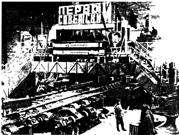
Пуск первого советского блюминга, изготовленного на Ижорском заводе, в новом прокатном цехе №1 Макеевского металлургического завода, г. Макеевка, 1933 г.
