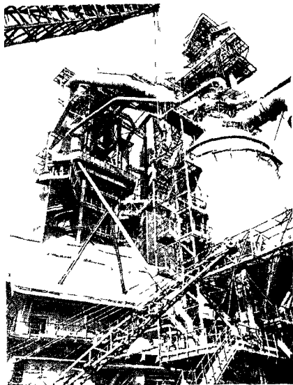
Домна «Косомольская» Ждановского металлургического завода им. С. Орджоникидзе «Азовсталь», г. Жданов Сталинской обл. 1958 г.
