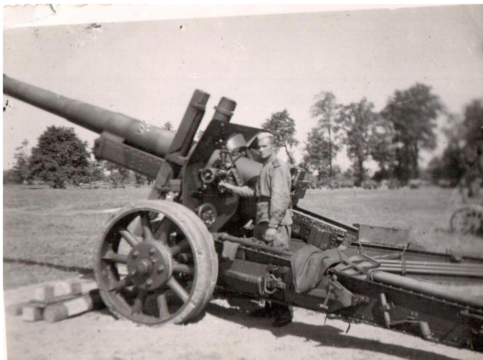
Тяжёлая 152 мм гаубица-пушка образца 1937 г. (МЛ-20) с колёсной базой от пушки образца 1910/34 гг.
