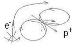
атом водорода
