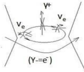
модель электрона
