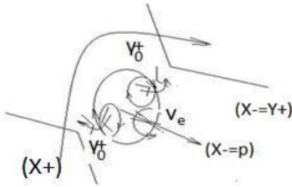
модель протона
