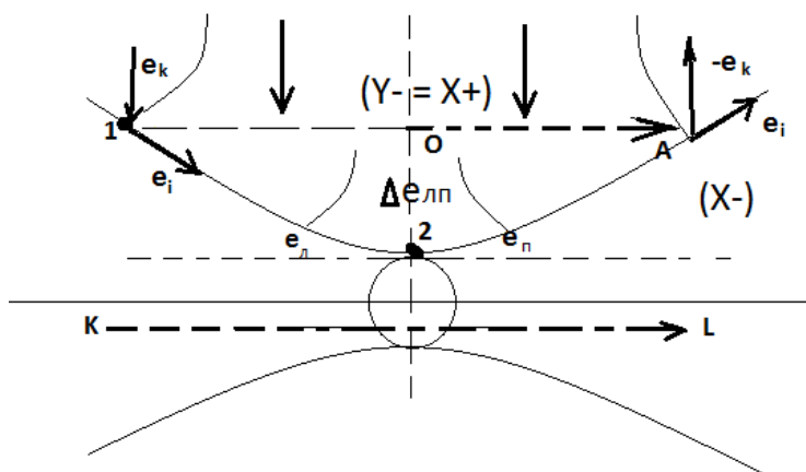
Точка (2) приводится к Евклидовому пространству сферы, где (e_i \perp e_k) и (e_i * e_k = 0) . Поэтому в окрестности точки (2) выделяем векторы (e_{\text{л}}) и (e_{\text{п}}) и берем среднее значение \Delta e_{\text{лп}} = \frac{1}{2} (e_{\text{л}} + e_{\text{п}}) .
