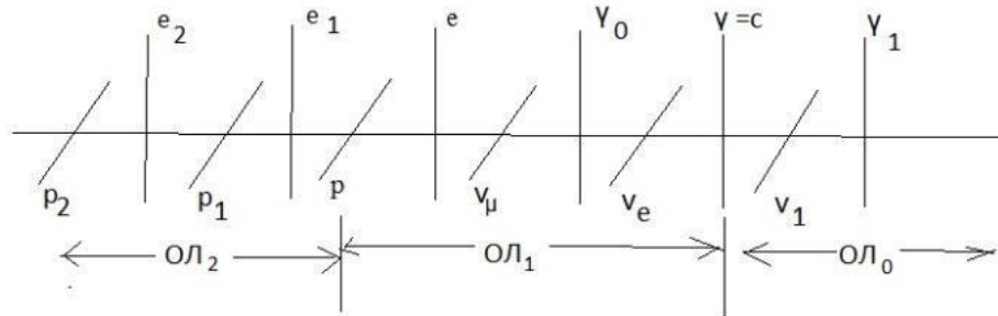
Рисунок 4. Неделимые кванты пространства-материи.
