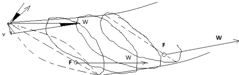
Рисунок3а. движение Земли вокруг Солнца по эллипсу с прецессией 23,5^0
