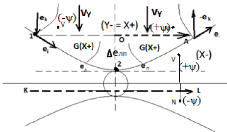
Рисунок 7. Квантовое гравит( X^+ = Y^- ) массовое поле.
