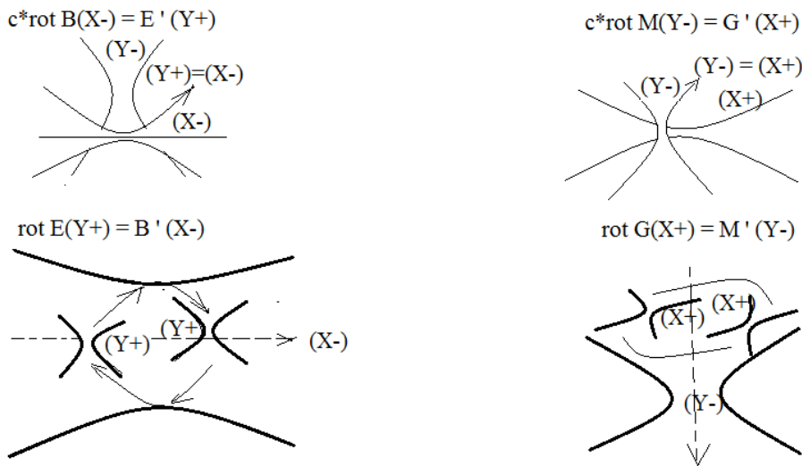
Рисунок 2.2-2. Единые поля пространства-материи
