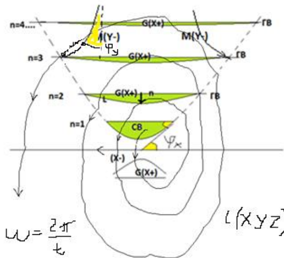
Рисунок 3.2 Квантовые гравитационные поля.
