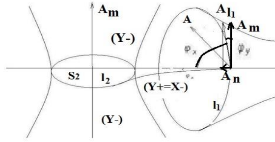
Figure 2.2-1. электро(Y+ = X-) магнитные и гравит(X+ = Y-) массовые поля.
