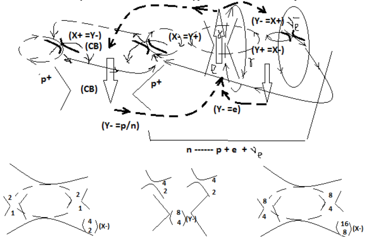
Figure 6.3 Квант ( Y- = p/n ) и аналогично ( Y- = 2n ) Сильного Взаимодействия Исходя из этих свойств ( X- = p^+ ) и ( X- = \nu_e^- ), время распада нейтрона в сильном ( X- ) магнитном поле должно измениться. Это проверяется в эксперименте.
