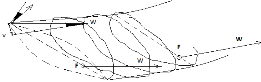
Figure 3.4. движение Земли вокруг Солнца по эллипсу с прецессией 23,5°
