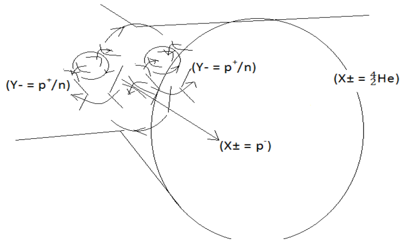
Рисунок 5.3 модель синтеза
