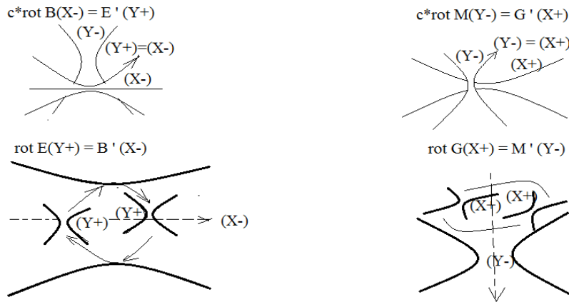
Figure 2.2. Единые поля пространства-материи
